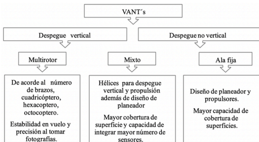
Figura 1. Clasificación de los VANT's y su utilidad de acuerdo con su diseño.
